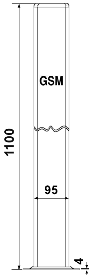
Frontansicht
