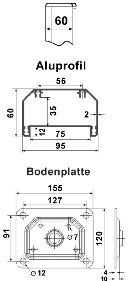
Seitenansicht
